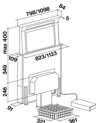
Versione filtrante (motore Slim) con filtro Carbon.Zeo Sottobase small (KACL.930)
