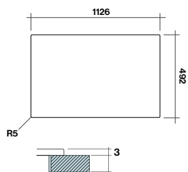
Dimensioni foro per installazione in appoggio (M3)
