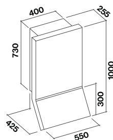
Versione h1000
