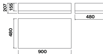
Versione Parete
