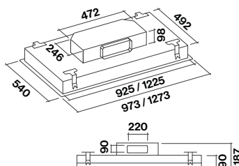
Motore Slim (solo su cappa)
