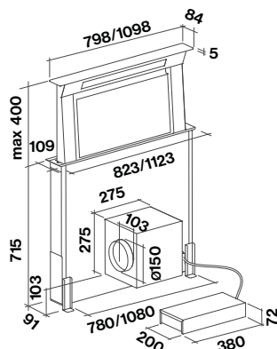
Versione aspirante (motore 950 m3/h montato su cappa)
