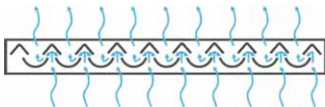
Profilo del filtro a lame incrociate con schema condensazione dei vapori.
