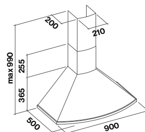
Versione parete
