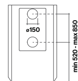
Vista posteriore
