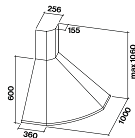
Versione angolo
