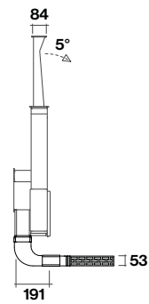
Vista laterale installazione con motore Slim posteriore, filtro sottobase KACL.951 (h 60 mm)
