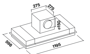
Motore sottotetto installato sulla cappa
