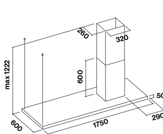
Versione Destra.
