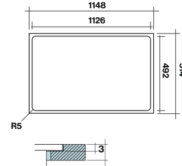
Dimensioni foro per installazione a filo (M3)
