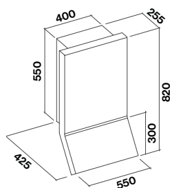
Versione h820
