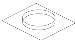
Flangia per motori e aspiratori ad alta potenza (1500 m³/h) KACL.396 ø200
