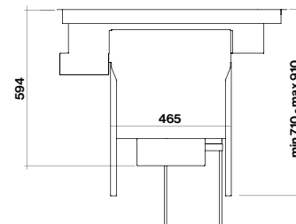
Vista frontale
