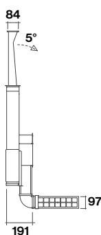
Vista laterale installazione con motore Slim anteriore
