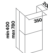
Camino opzionale
