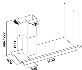
Versione Sinistra.
