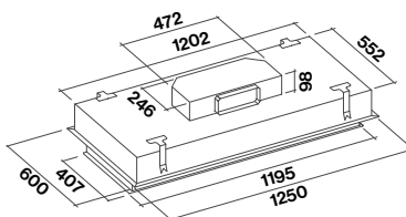
Motore Slim (solo su cappa)
