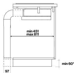
Tutte le versioni: Vista laterale
