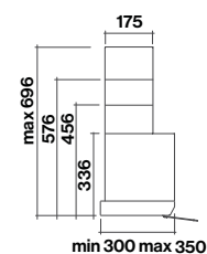
Vista posteriore
