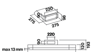
Unità remote
