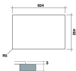
Dimensioni foro per installazione in appoggio (M1 / M2)
