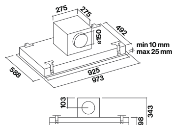
Motore Slim (solo su cappa)
