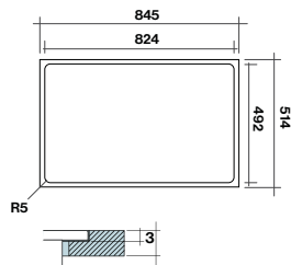
Dimensioni foro per installazione a filo (M1 / M2)
