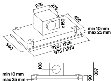
Motore sottotetto installato sulla cappa
