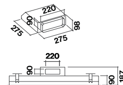
Raccordo (KACL.789)
