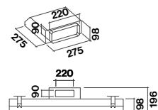
Raccordo (KACL.789)
