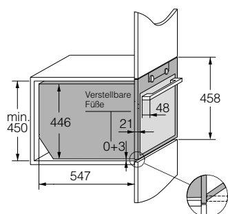
Abmessungen des Gerätes
