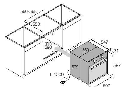
Unterschrankeinbau Anschluss 230 V oder 400 V (siehe Seite 231)
