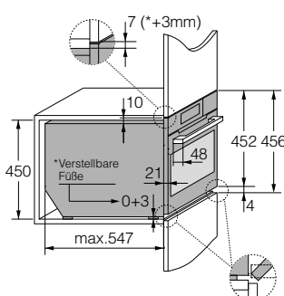
Abmessungen des Gerätes
