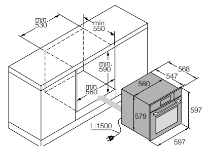
Unterschränkeinbau Anschluss 230 V oder 400 V (siehe Seite 231)
