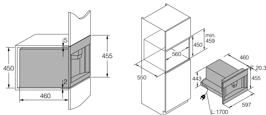
Abmessungen des Gerätes
