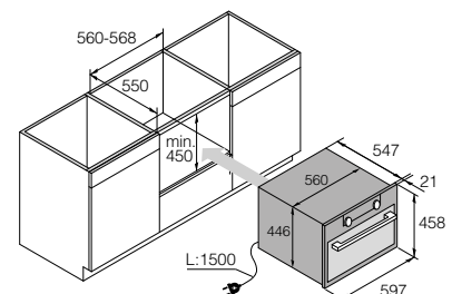
Unterschrankeinbau
