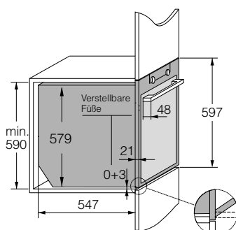
Abmessungen des Gerätes
