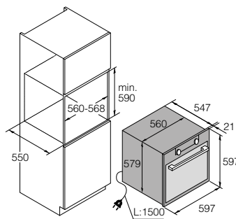
Hochschränkeinbau
