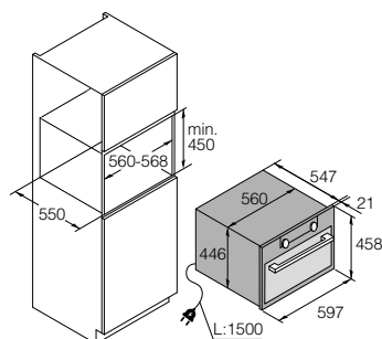
Hochschrankeinbau
