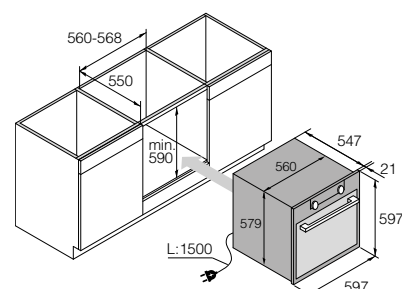
Unterschrankeinbau Anschluss 230 V oder 400 V (siehe Seite 231)
