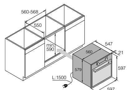
Unterschränkeinbau Anschluss 230 V oder 400 V (siehe Seite 231)
