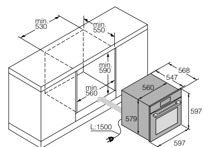
Unterschrank einbau Anschluss 230 V oder 400 V (siehe Seite 231)
