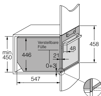
Abmessungen des Gerätes
