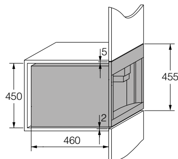
Abmessungen des Gerätes
