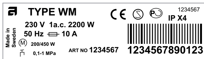
Exemple de plaquette signalétique
