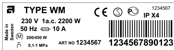
Esempio di targhetta dei dati
