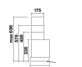
Vista laterale con camini opzionali
