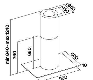
Versione Isola con vetro (opzionale)
