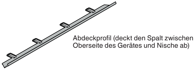
Abdeckungen Montage links oben bei Türanschlag rechts. Montage rechts oben bei Türanschlag links.
