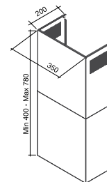
Schachtverlängerung Wandhaube / Rallonge cheminée pour hottes murales / Camino opzionale
