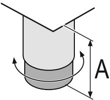
Fig. 14 Il piedino è regolabile da A = 115 mm (4 1/2 in) a 175 mm (6 7/8 in).*
